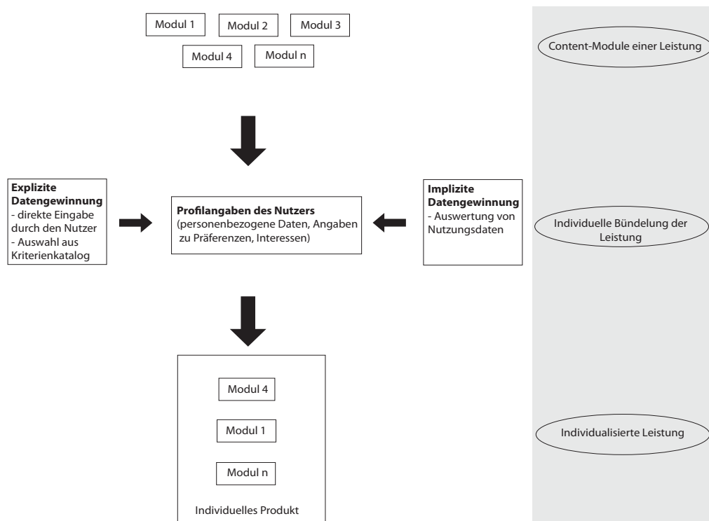
Abbildung 5: Individuelle Produktkonfiguration
