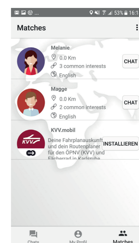
Abb. 2: Matches/Werbung
