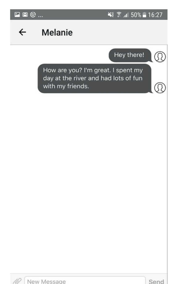
Abb. 3: Live Chat
