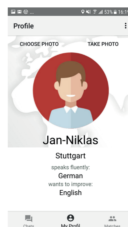
Abb. 1: Benutzerprofil
