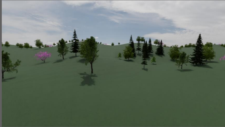
Umgebung, HDRI
